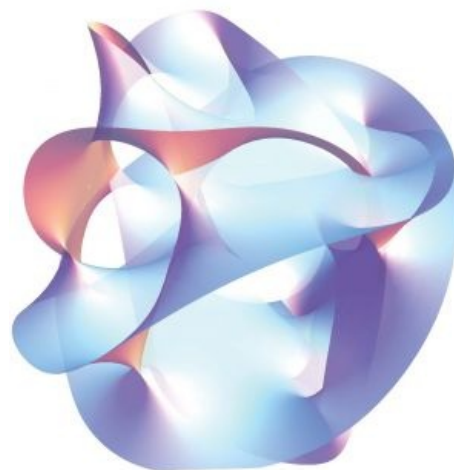
Двумерная проекция трехмерной визуализации пространства Калаби-Яу
